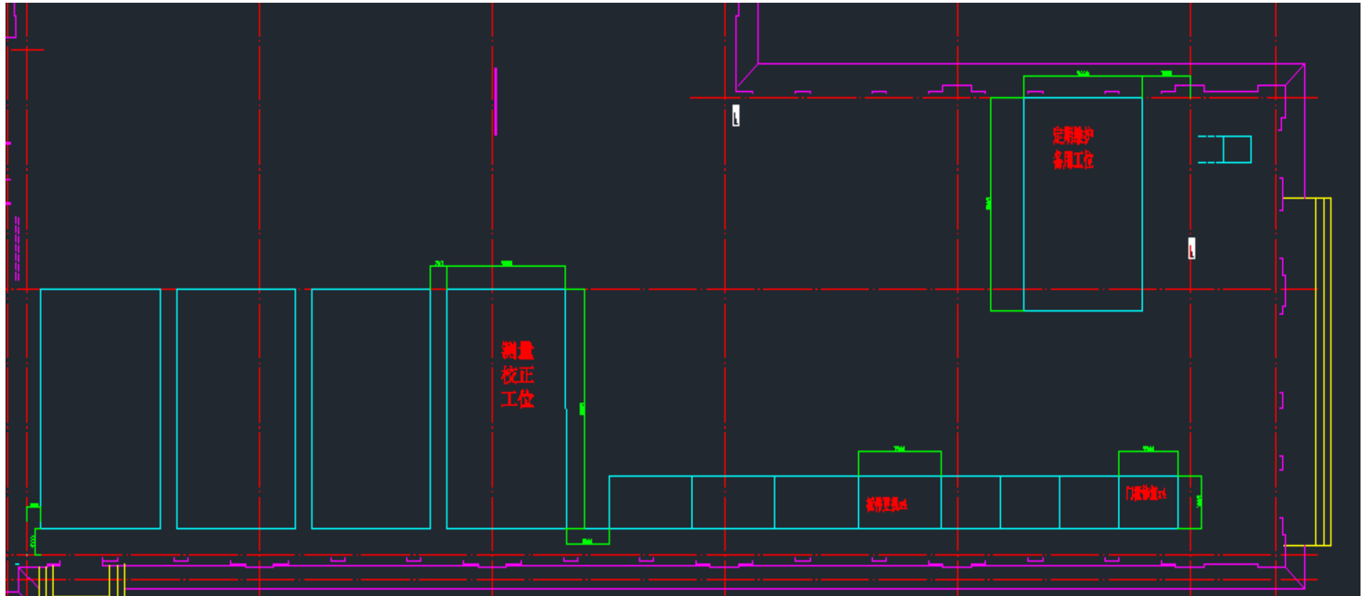
钣金工位布置图
